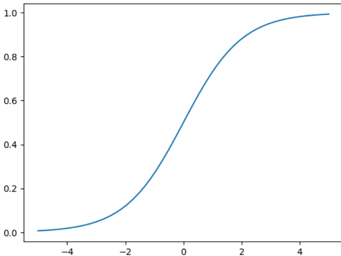
Figura 2.2 Grafico della funzione sigmoidea con matplotlib.
