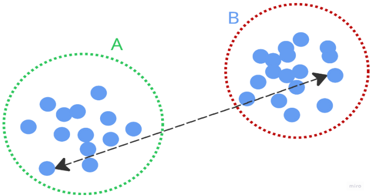
Figura 1.4 In questa figura è rappresentato il metodo di collegamento completo in cui i punti colorati in blu sono i punti dati e la freccia rappresenta la distanza massima tra due punti di cluster diversi.
